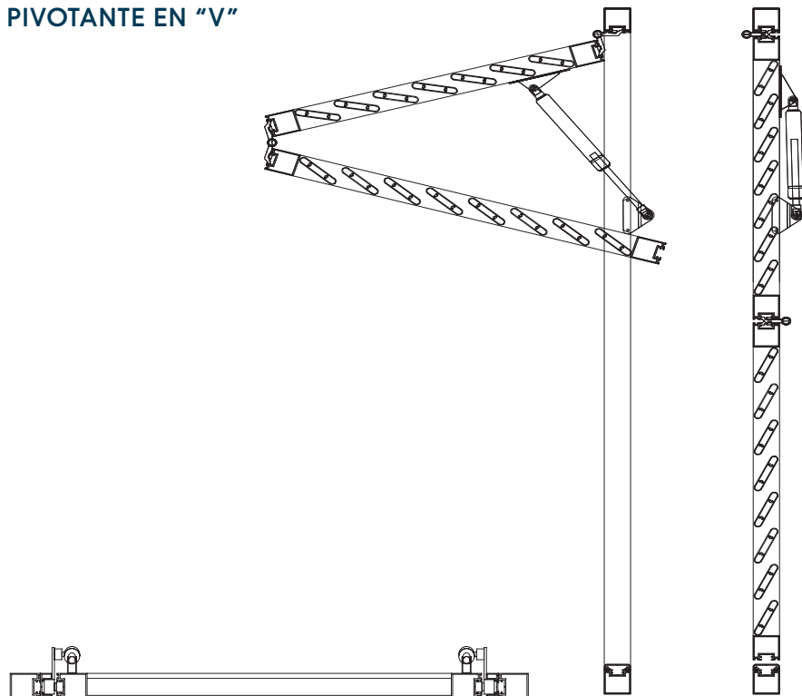
ACTUADORES OLEONEUMÁTICOS
