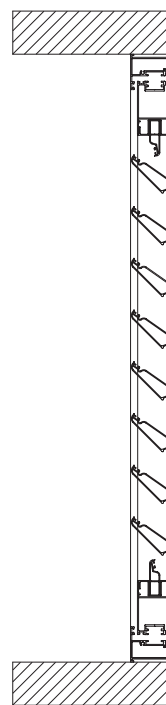
MARCO CON SOLAPE
