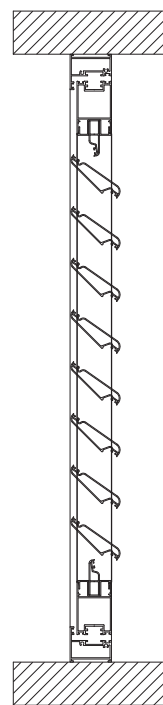
MARCO SIN SOLAPE
