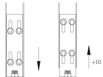
Soportes inoxidables con regulación vertical del poste.
