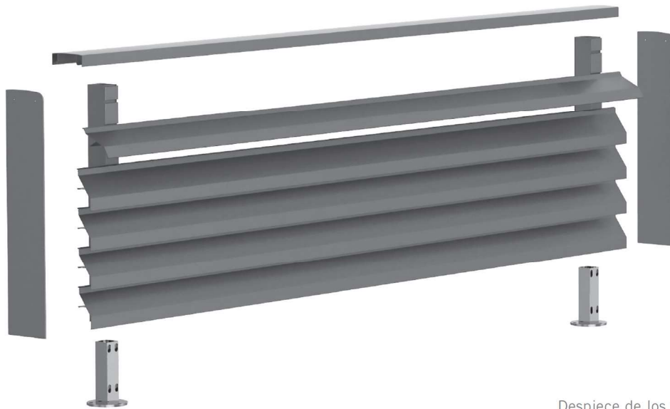
Despiece de los principales elementos del sistema.
